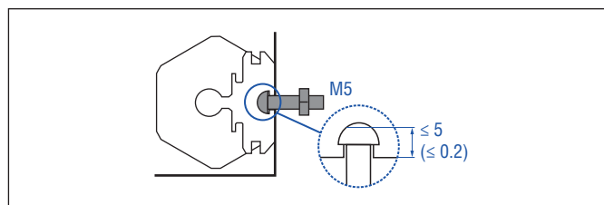
Fig. 11: T-slot nut M5 (part no. 401 602)
