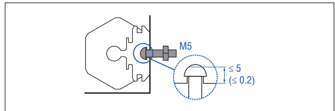
Fig. 11: T-slot nut M5 (part no. 401 602)
