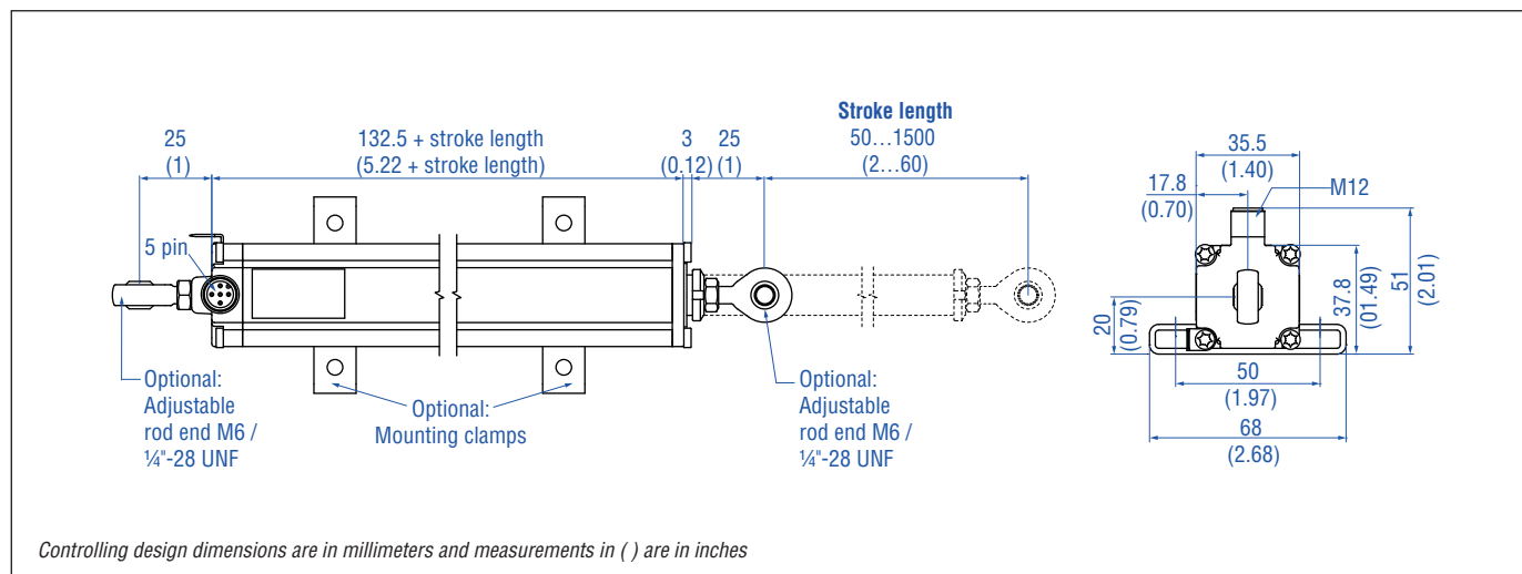
Fig. 3: Temposonics® ER
