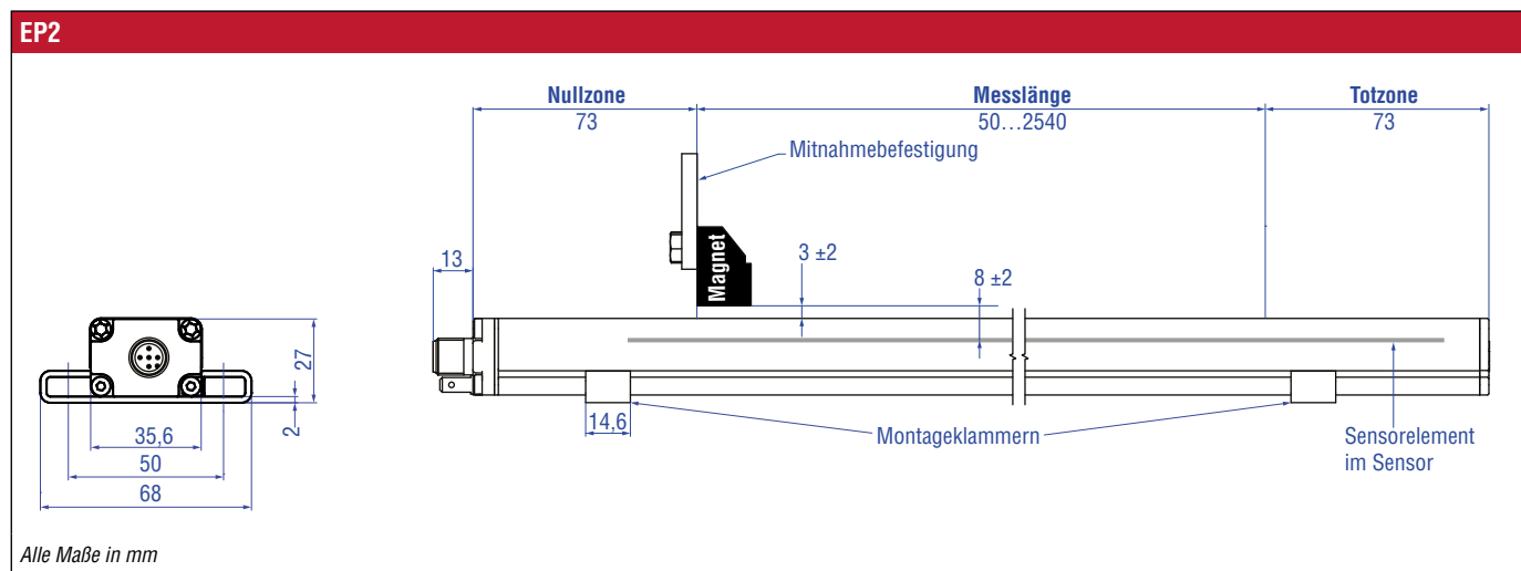
Abb. 3: Temposonics® EP2 mit Blockmagnet
