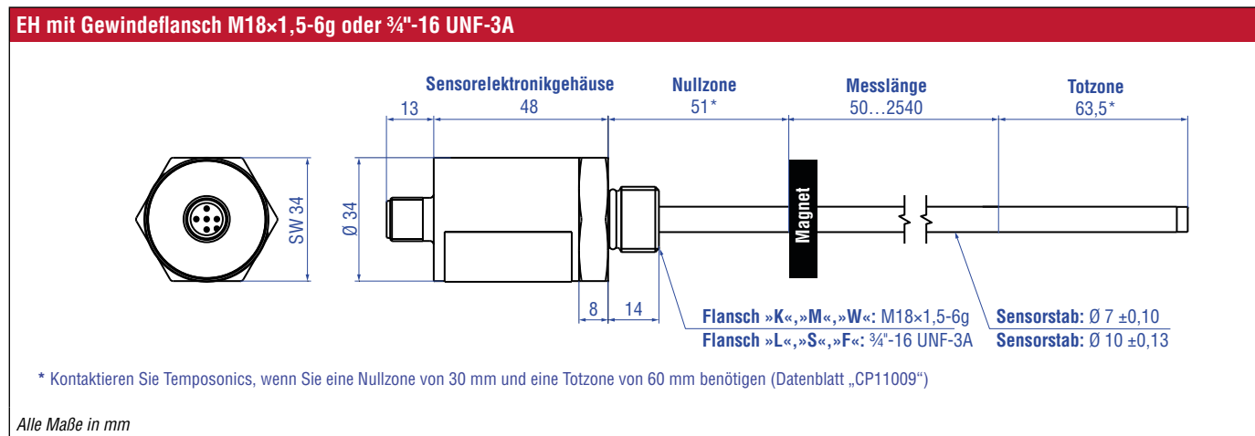
Abb. 3: Temposonics® EH mit Ringmagnet
